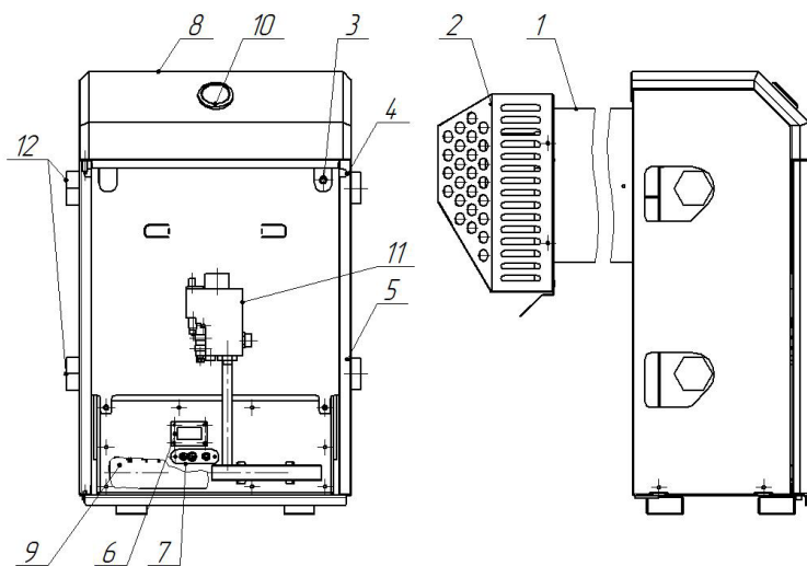
Рисунок 2 Устройство изделия
