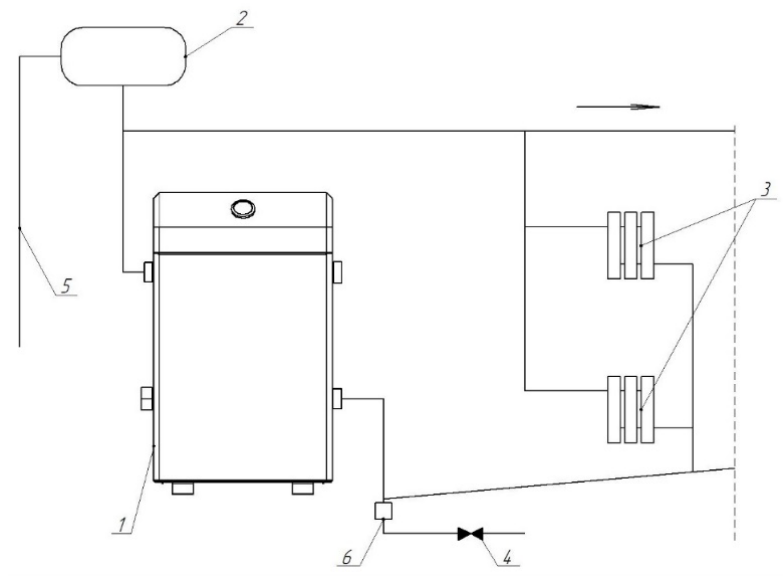
Рисунок 5 Примерная схема открытой системы отопления *
