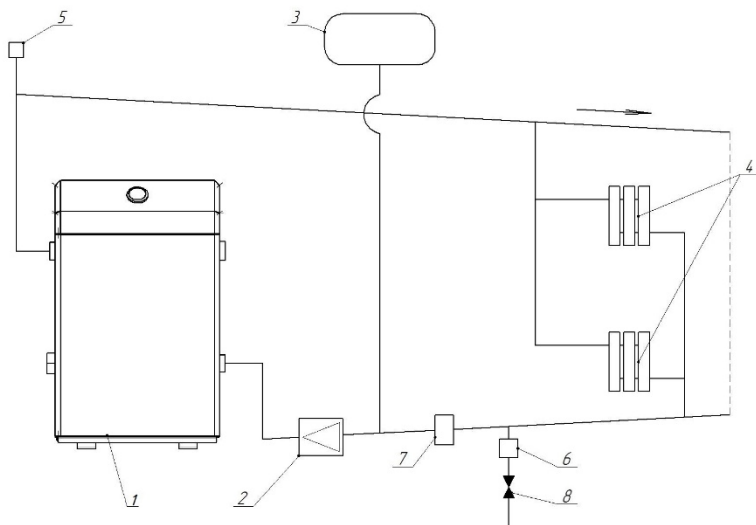
Рисунок 6 Примерная схема открытой системы отопления с циркуляционным насосом *
