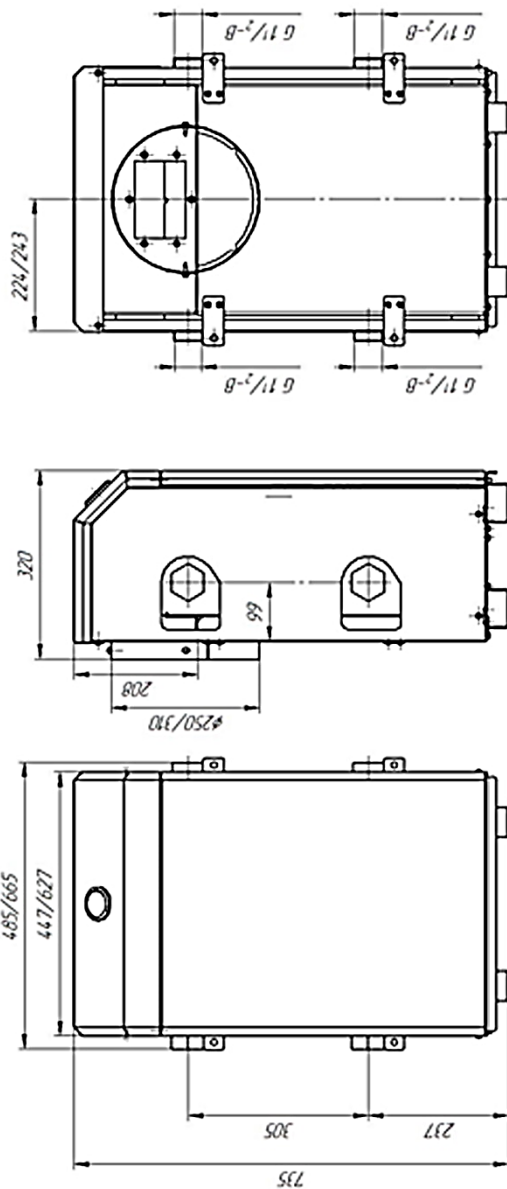
Рисунок 1 Присоединительные размеры котла мощностью 7,5-10 кВт/12,5-16кВт
