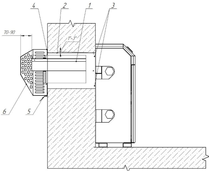
Рисунок 3 Монтаж котла
