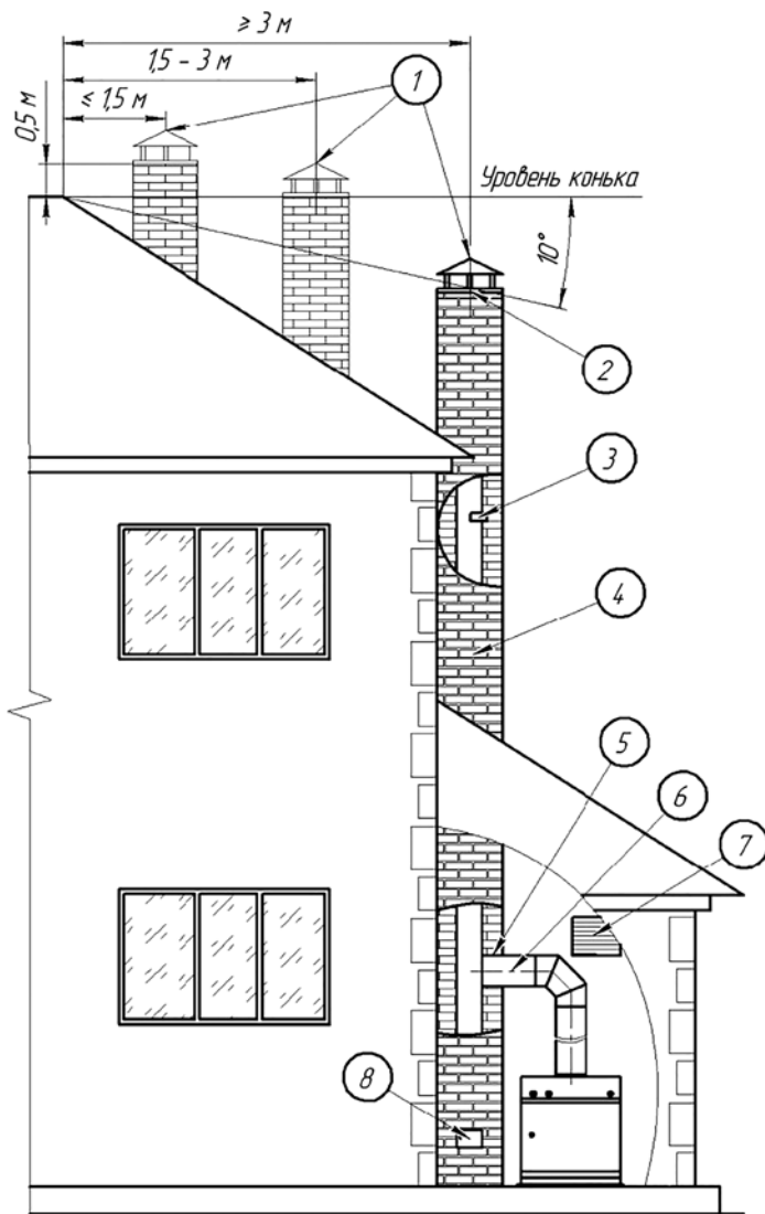
Рисунок 7. Основные причины неудовлетворительной тяги.
