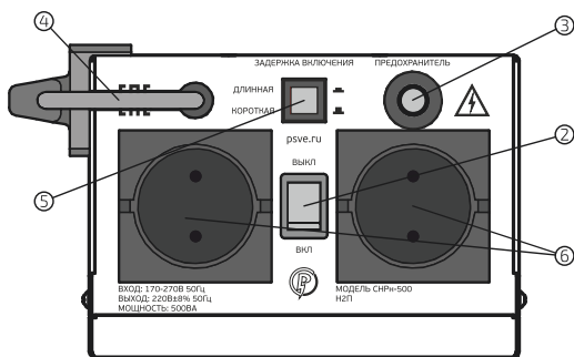
Рисунок 2. Вид сверху
