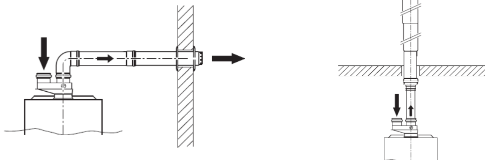
Рис.6 Дымоудаление типов В
