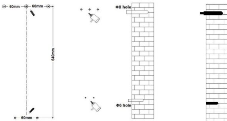
Рис. 5. Монтажные размеры крепежных отверстий
