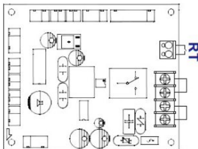
Рис. 9 Схема подключения комнатного термостата
