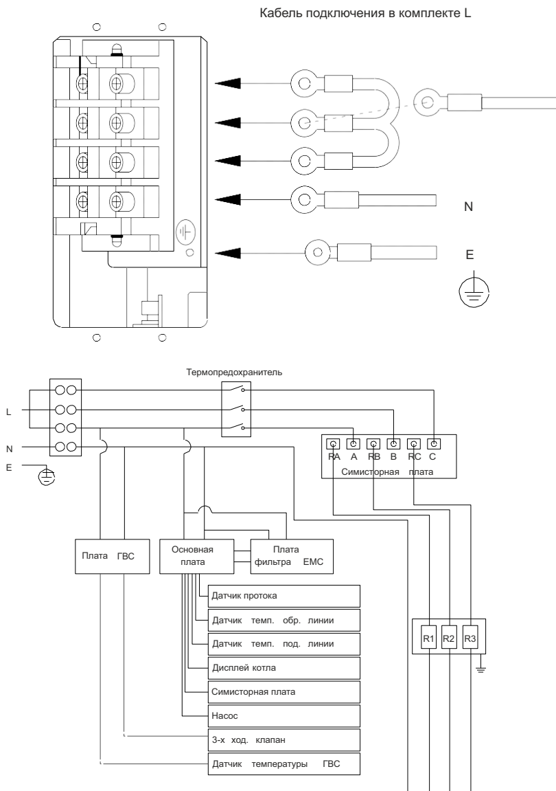
Рис. 7. Схема однофазного подключения
