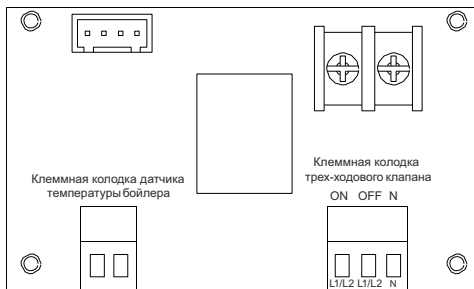
Рис. 10 Схема подключения трехходового клапана и датчика температуры бойлера
