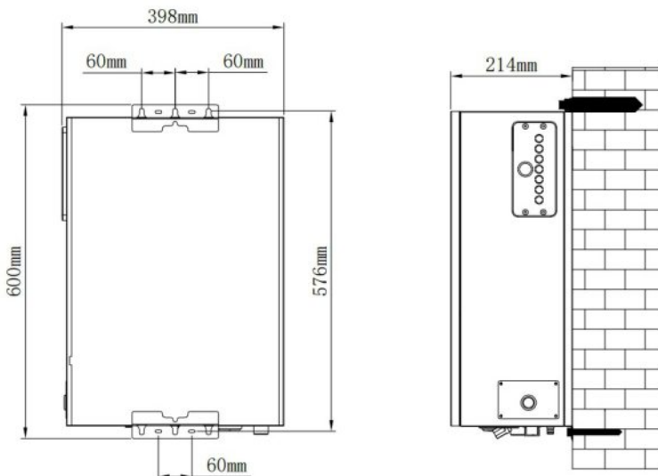
Рис. 4. Размещение прибора
