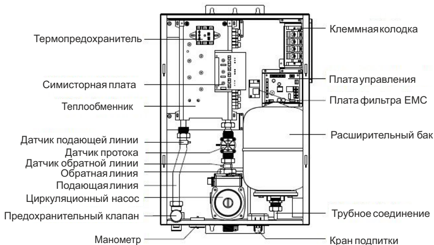
Рис. 1. Конструкция изделия
