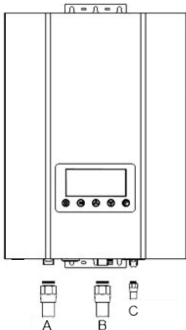
Рис. 6 Гидравлическое подключение котла
