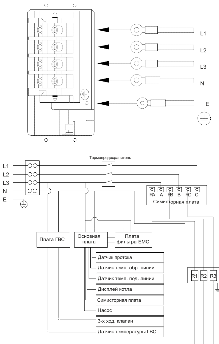
Рис. 8. Схема трехфазного подключения
